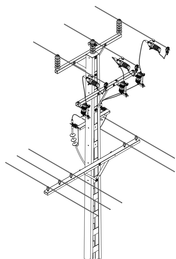
ISOMETRIC VIEW N.T.S.
