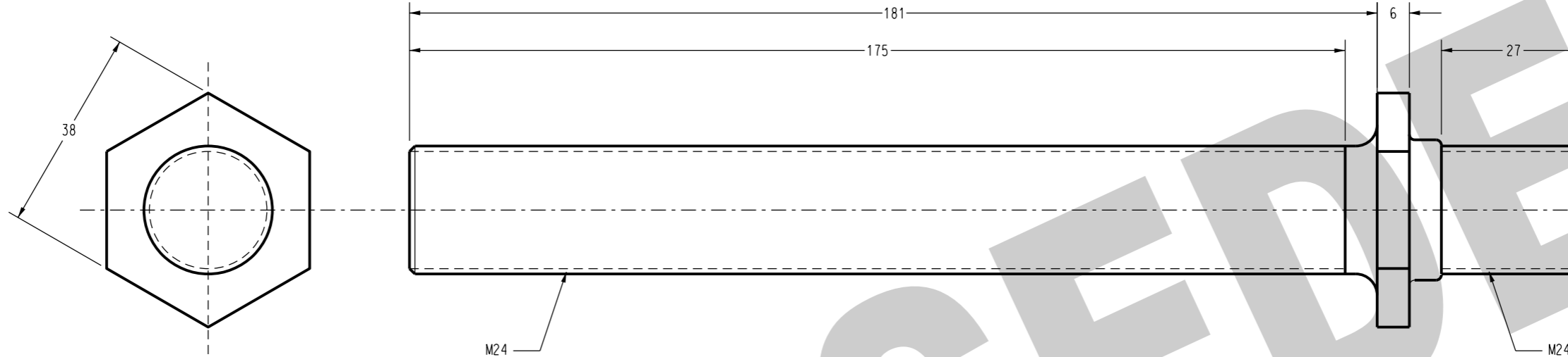
ITEM 1: INSULATOR STUD
