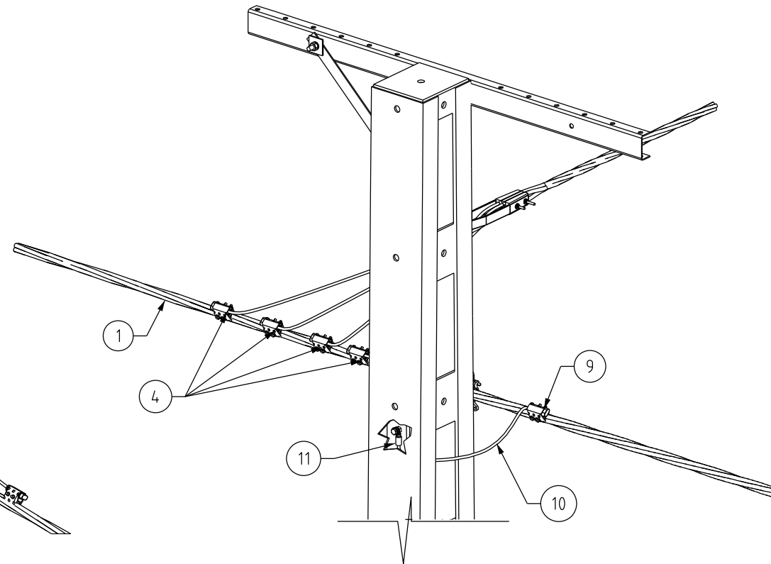
ISOMETRIC BACK VIEW SCALE N.T.S.
