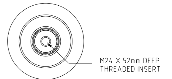
DETAIL A: BASE
