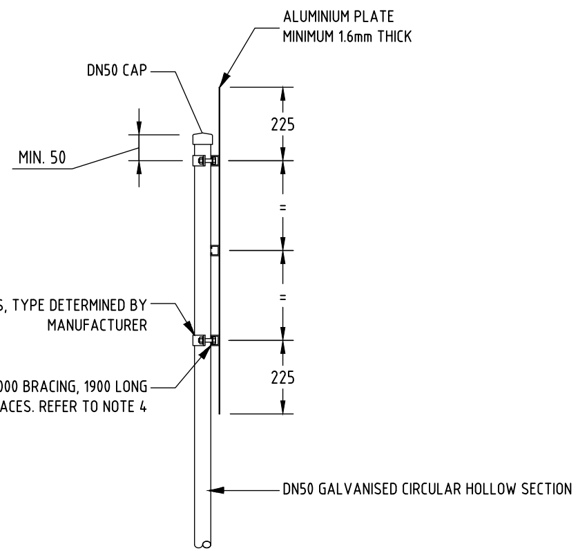
SECTION A-A
