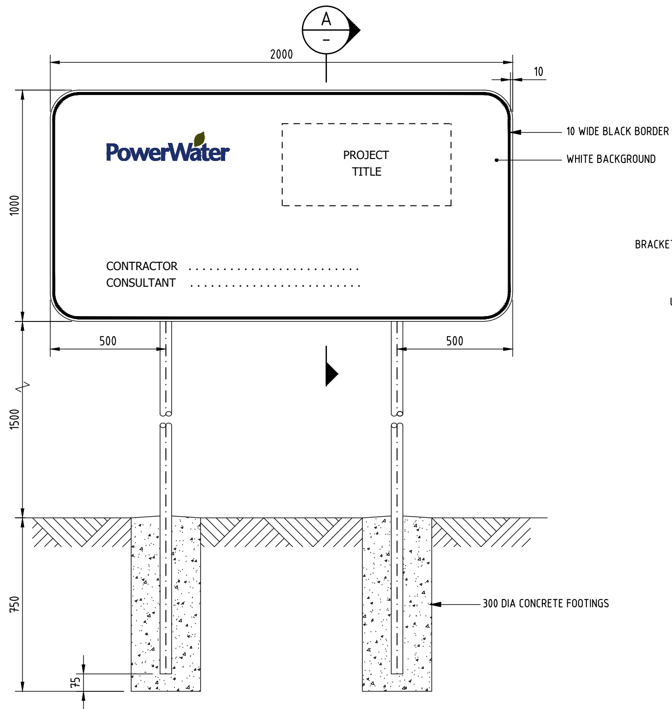
ELEVATION
