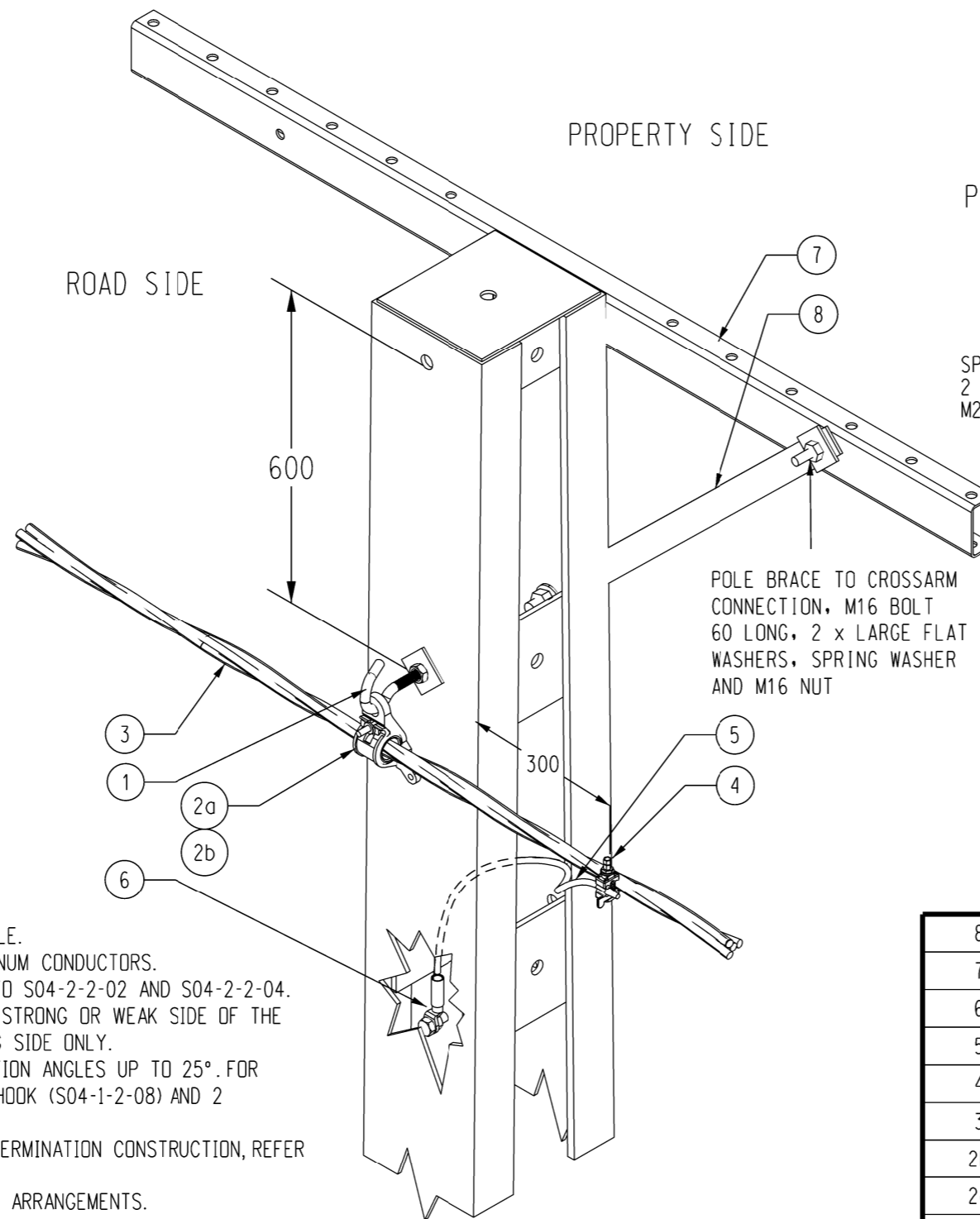
ISOMETRIC VIEW FRONT N.T.S.
